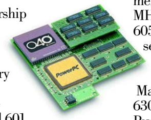
PowerCard 601
